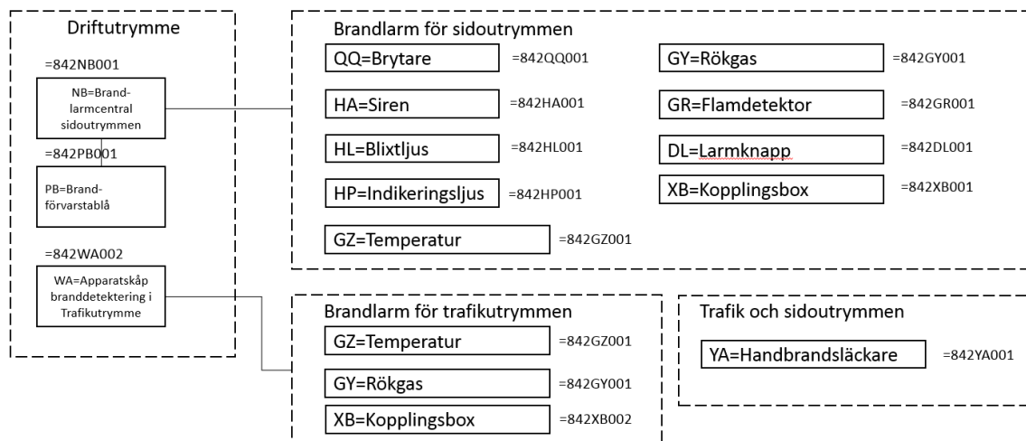
Figur 5.9.4.8 Kravprincip för Brandlarmssystem.
