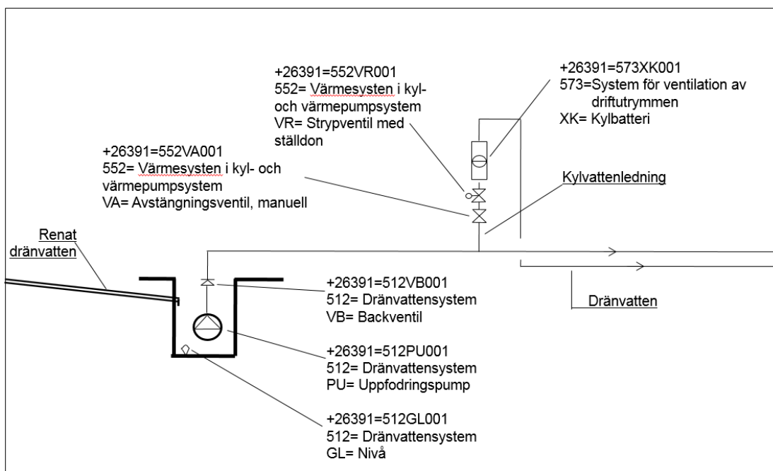
Figur 5.6.3.1 Kravprincip för Pumpstation med dränvatten och kyla.
