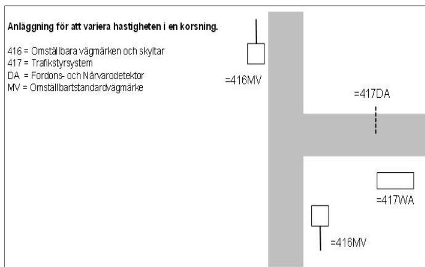
Figur 5.5.3.7. Kravprincip för korsning med varierande hastighet.
