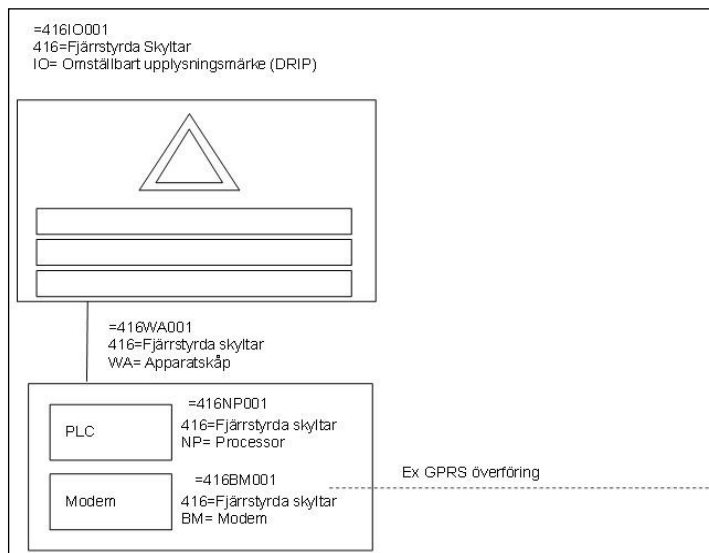
Figur 5.5.3.6. Kravprincip för fjärrstyrd skylt typ DRIP.
