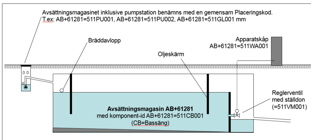
Figur 5.6.3.2 Kravprincip för Avsättningsmagasin med Pumpstation.
