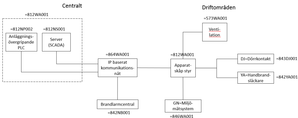
Figur 5.9.4.9 Kravprincip för anslutna systems relation till anläggningsövergripande styr- och övervakningssystem.
