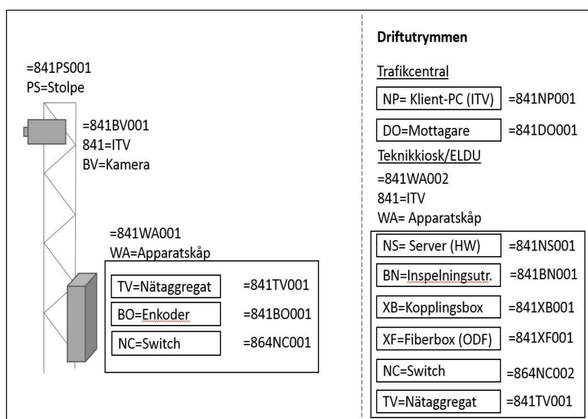
Figur 5.9.4.2 Kravprincip för ITV-system (841).
