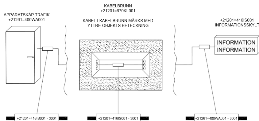
Figur 5.12.3 Kravprincip för kabelmärkning i kabelbrunn.
