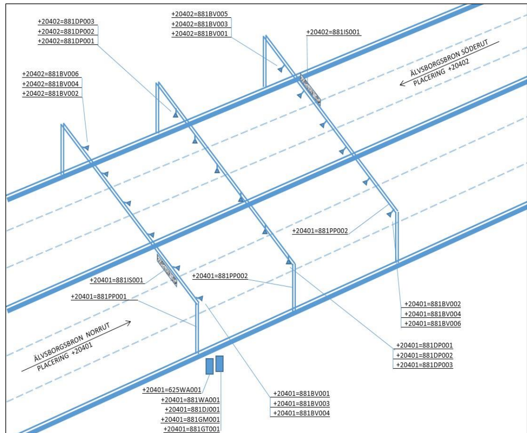
Figur 5.9.4.7 Kravprincip för 881 Avläsnings- och betalsystem.
