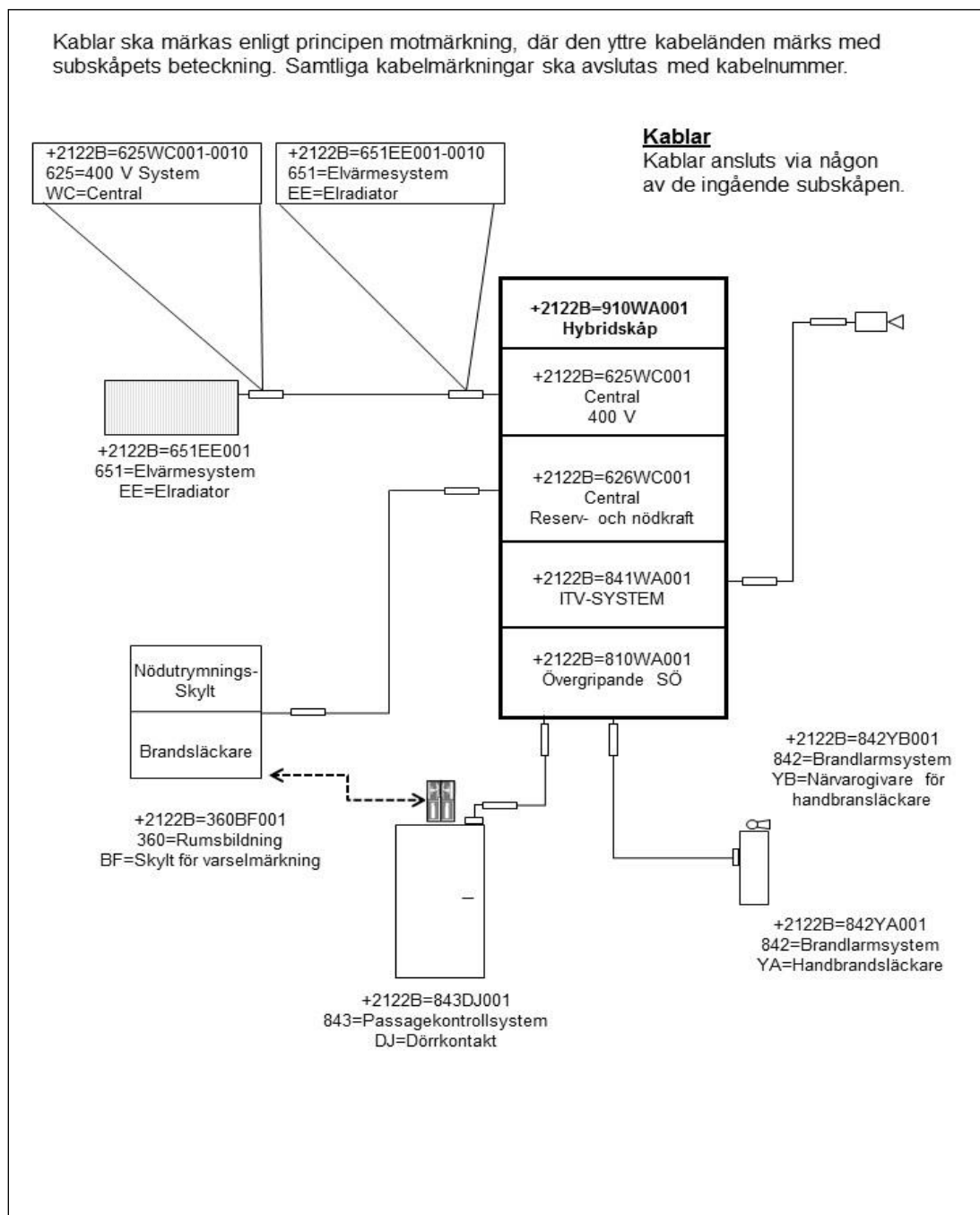
Figur 5.10.3 Kravprincip för kabelmärkning för hybridskåp.
