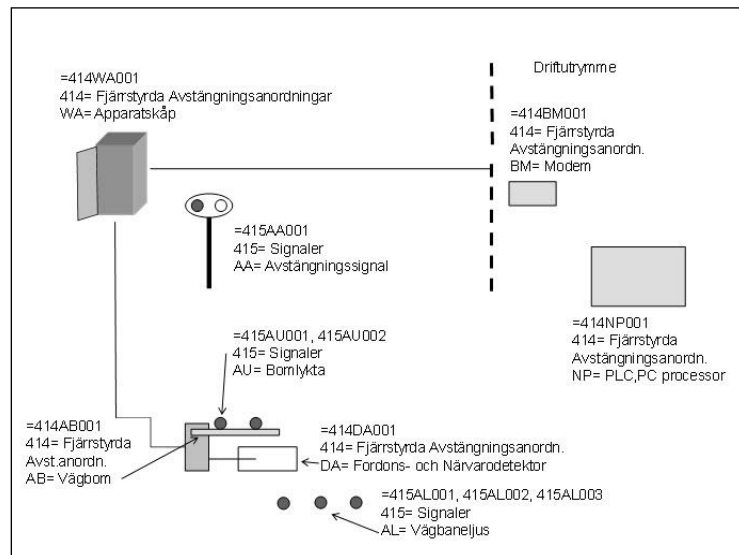
Figur 5.5.3.1 Kravprincip för fjärrstyrd bomanläggning.
