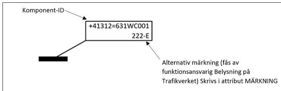
Figur 5.14-1 Krav på märkskylt med komponent-ID samt alternativ märkning på ritning.
