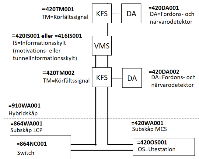
Figur 5.5.3.2-1. Kravprincip för MCS (MTM/2).
