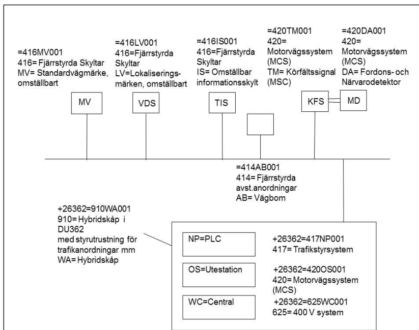
Figur 5.5.3.3. Kravprincip för Hybridskåp med fjärrstyrda skyltar.
