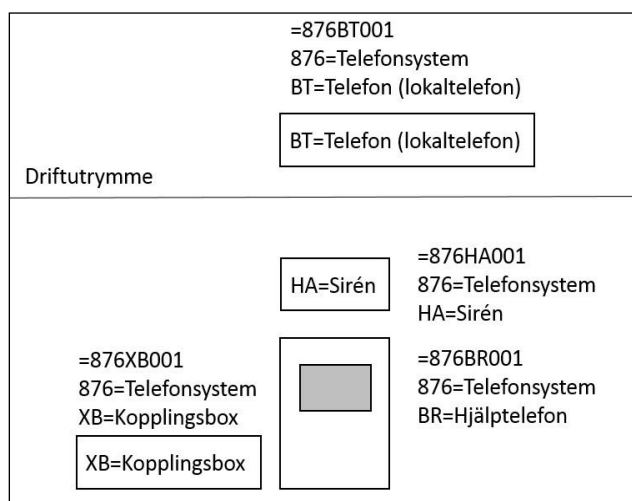
Figur 5.9.4.6 Kravprincip för Telefonisystem (876).
