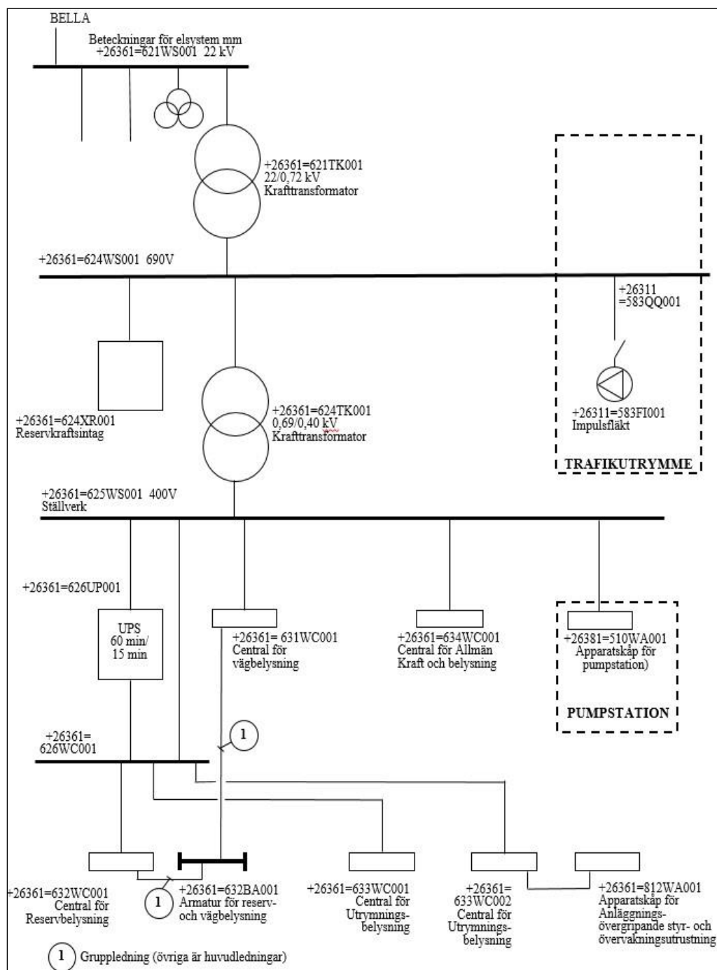
Figur 5.7.4-3 Kravprincip för systemhierarki för EI i tunnel.
