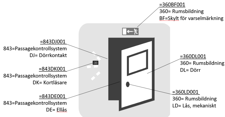
Figur 5.4.3 Kravprincip för dörrkomponenter.
