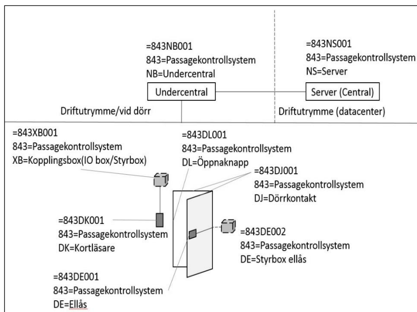
Figur 5.9.4.3 Kravprincip för Passersystem (843).
