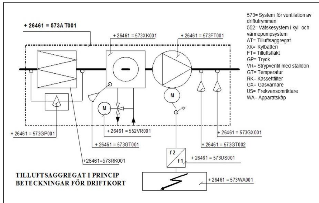
Figur 5.6.6 Kravprincip för tilluftsaggregat.
