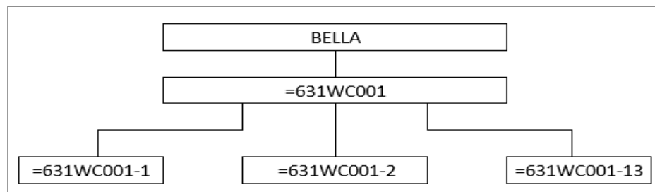
Figur 5.11.2-2 Kravprincip för belysningscentral med tre anslutande grupper.
