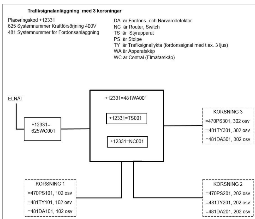
Figur 5.5.3.8. Kravprincip för korsning med tre trafiksignaler.
