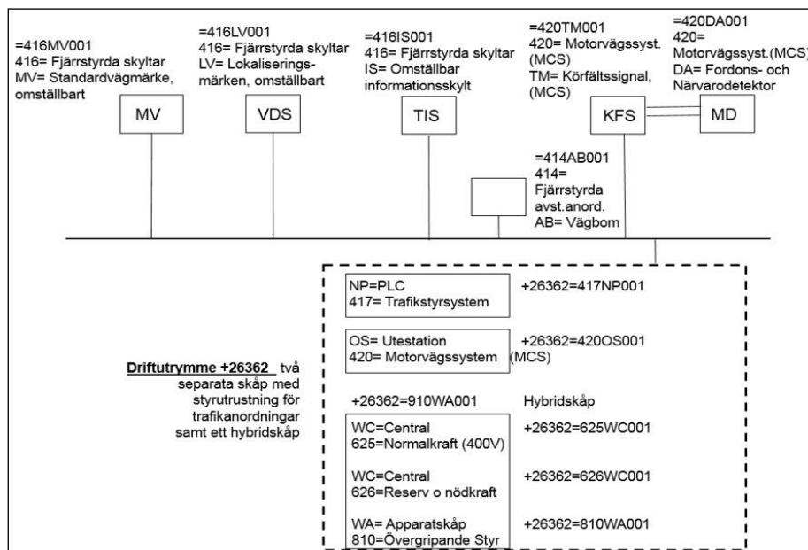
Figur 5.5.3.4 Kravprincip för två apparatskåp samt hybridskåp och fjärrstyrda skyltar.
