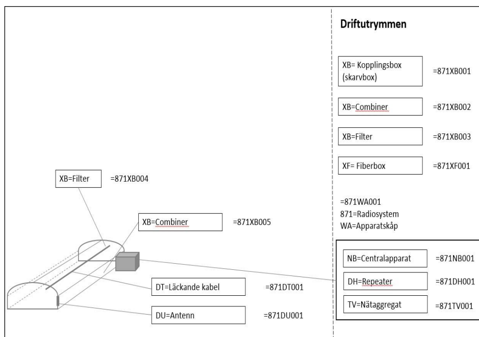
Figur 5.9.4.4 Kravprincip för Radiosystem (871).
