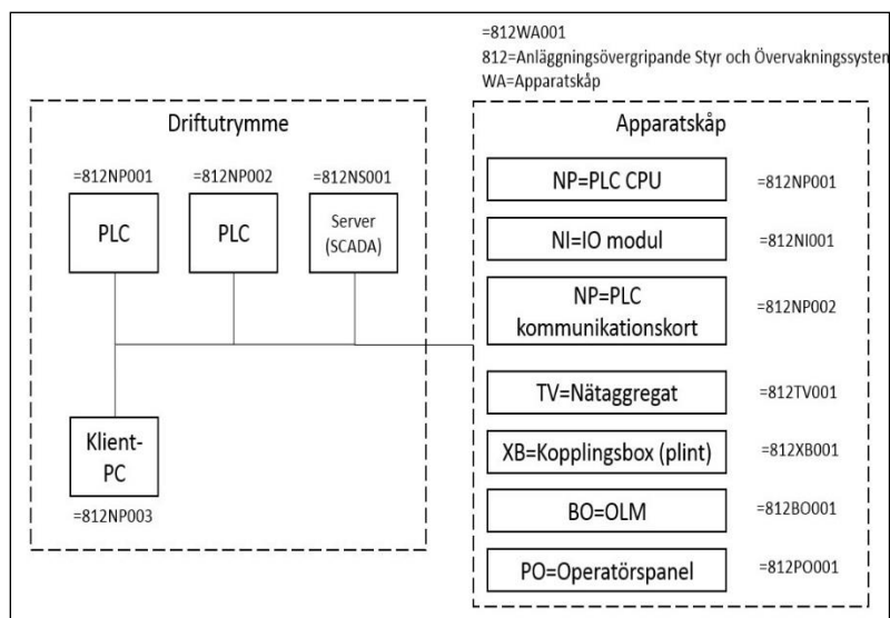
Figur 5.9.4.1 Kravprincip för Anläggningsövergripande styr och övervakning (812).
