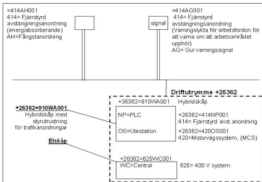
Figur 5.5.3.5 Kravprincip för apparatskåp placerat i driftutrymme.
