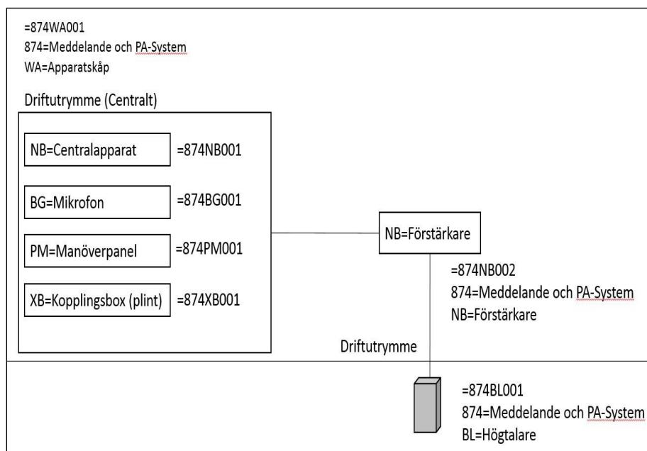
Figur 5.9.4.5 Kravprincip för Meddelandesystem och PA (874).
