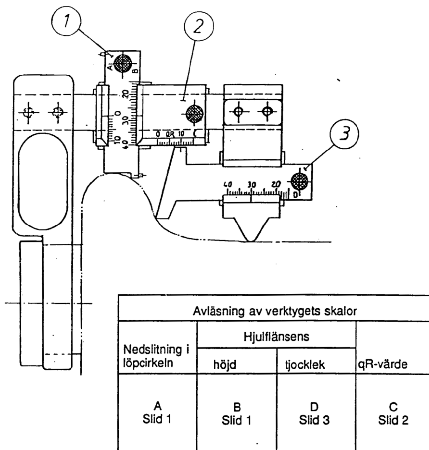
Figur 1: Mätton för hjulförlitning (art nr 86 15 9032 ME-20292)
