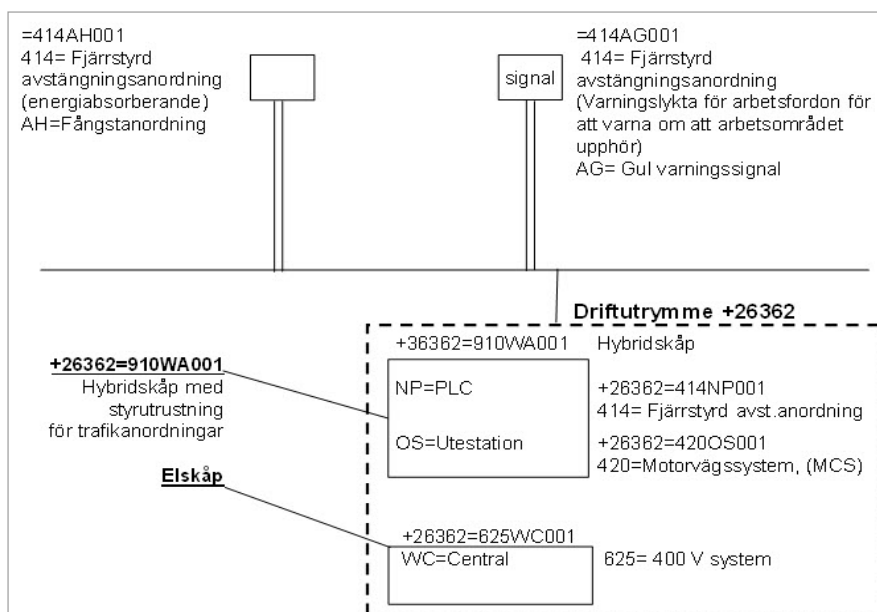
Figur 4.5.3.5 Kravprincip för apparatsskåp placerat i driftutrymme.
