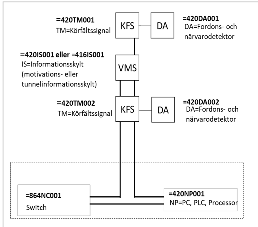
Figur 4.5.3.2-3. Kravprincip för Körfältssignal, tunnelinformations- eller motivationsskylt på gemensam skyltbärare (MTM/2 konverterad till LASSY)
