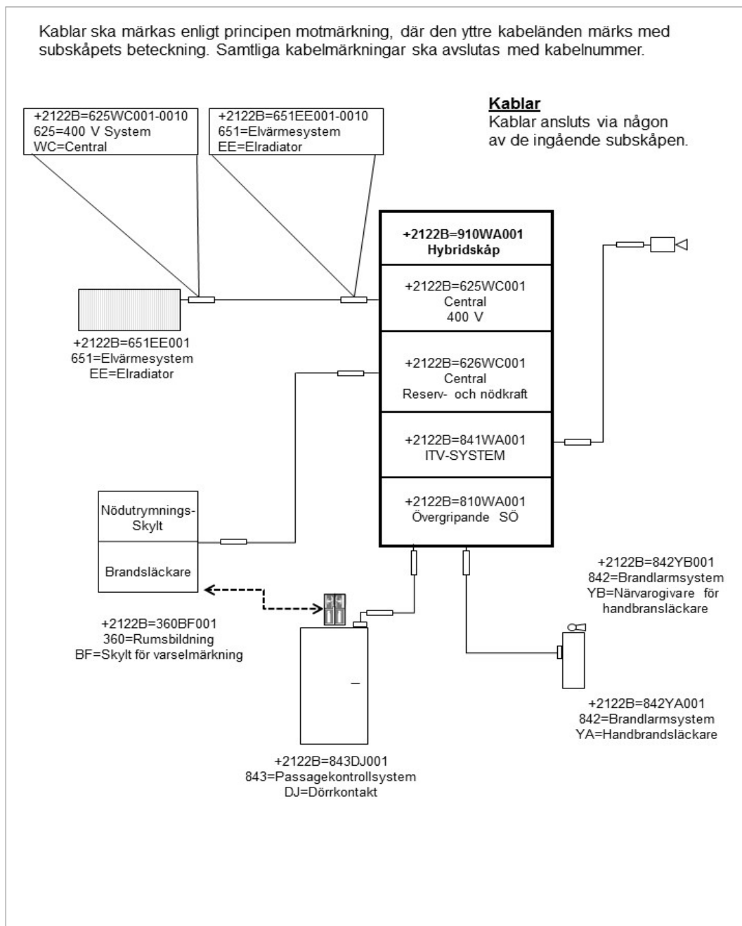
Figur 4.10.3 Kravprincip för kabelmärkning för hybridskåp.
