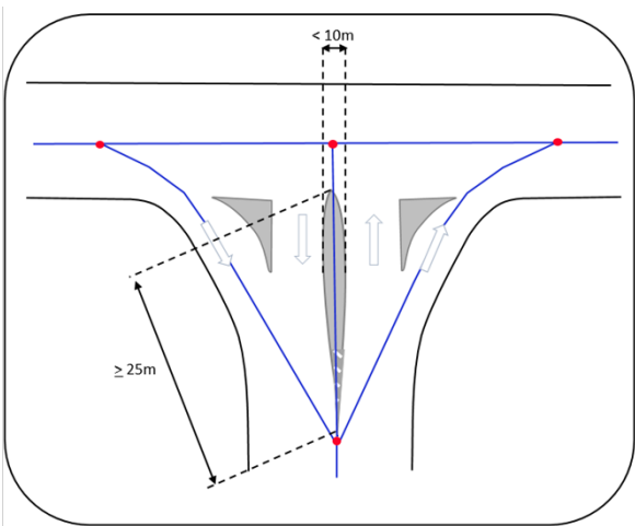
Figur 50 Riktningsgivande refug skapar separata länkar till höger och vänster. Mittrefug för smal för att dela upp länk.
