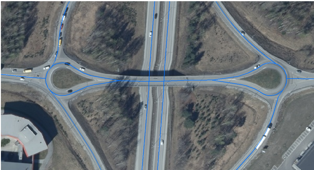
Figur 38 Exempel på "droppe".
