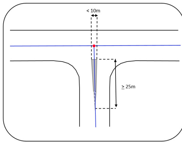
Figur 47 Ena sidan av refugen är mer än 25 meter, den kortaste sidan är mindre än 10 meter. Refugen skiljer trafik med motsatt körriktning.
