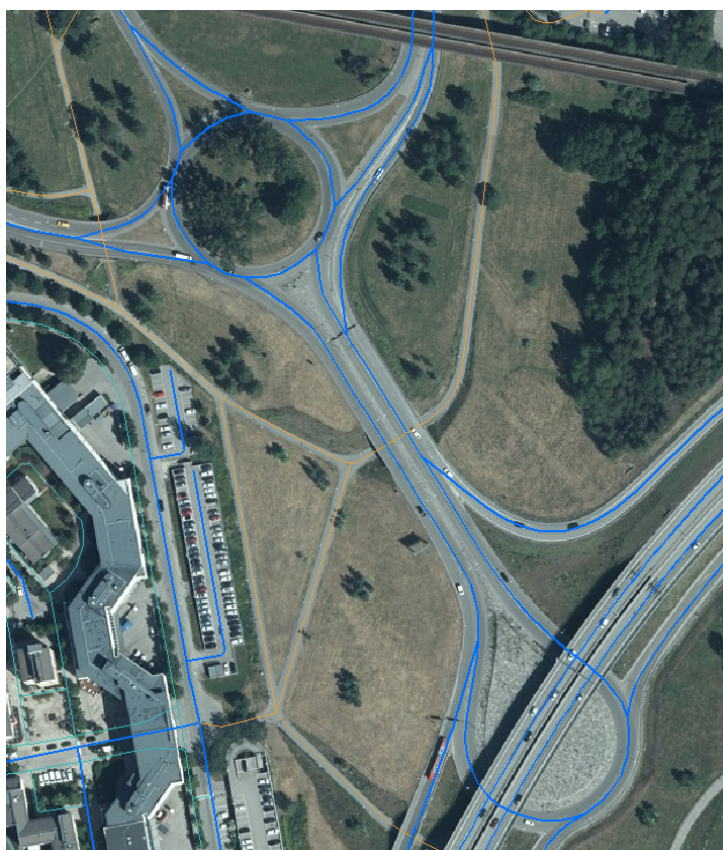
Figur 40 Exempel på "droppe" med fysisk barriär.
