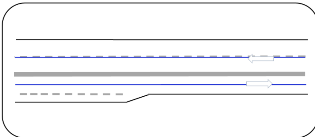
Figur 3 Korrekt placering av referenslinjerna vid en vägkombination av 2+2 och 2+1.
