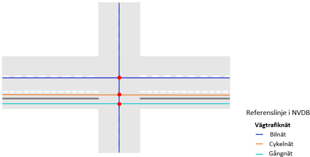
Figur 67 Bilden illustrerar hur ett cykelfält fortsätter över korsningen och övergångstället trots att vägmarkeringen för cykelfältet tillfälligt upphör.
