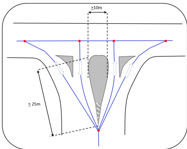
Figur 51 Alla refuger i korsningen uppfyller kravet på uppdelning av länkarna.
