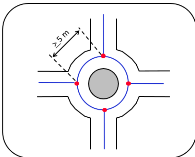
Figur 36 Cirkulationsplats (5 m gäller för avståndet mellan noder).
