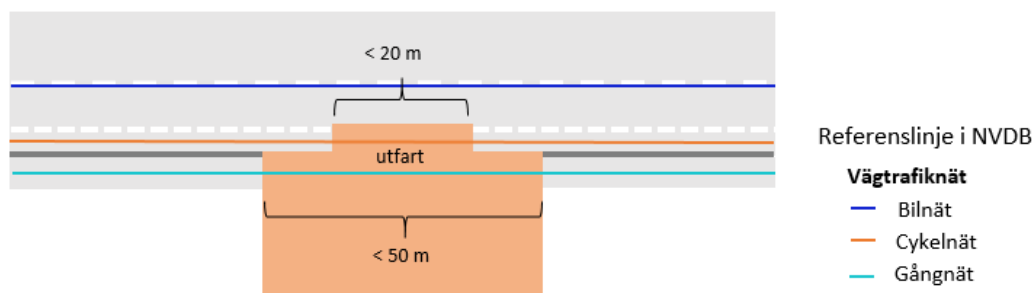
Figur 69 Enligt kontinuitetsregeln fortsätter cykelfältet över utfarten trots att vägmarkeringen för cykelfältet tillfälligt upphör. Motsvarande gäller för trottoaren där gångnätet fortsätter över utfarten trots att trottoar saknas.
