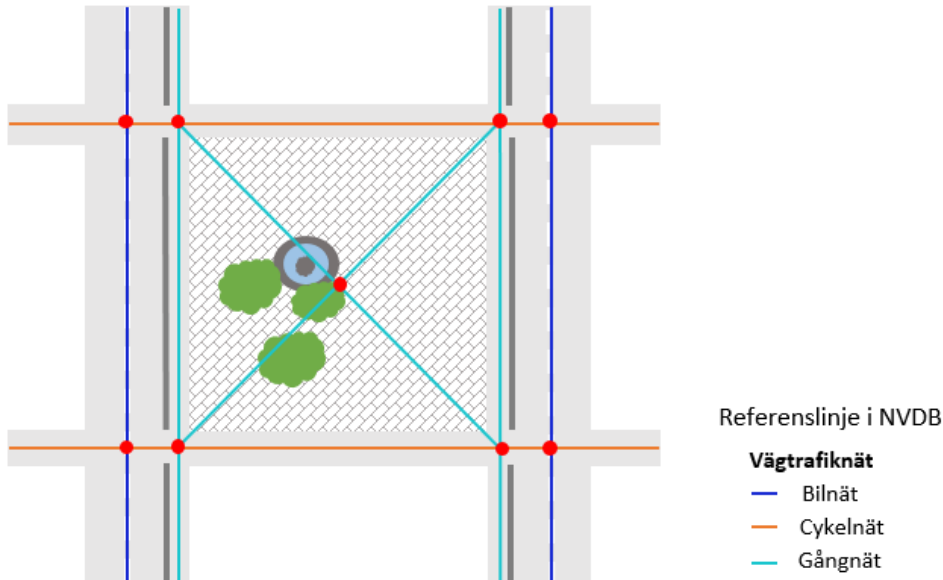
Figur 66 Exempel på gång- och cykelnät på öppna ytor t.ex. torg.
