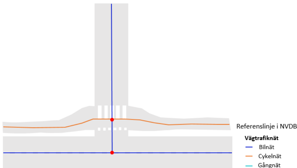
Figur 67 Gemensam referenslinje för gång- och cykelnät vid övergångsställe och cykelpassage.
