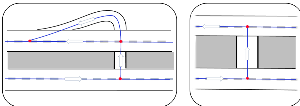
Figur 56 Två olika typer av driftvändplatser där tvärlänkar ska läggas till.
