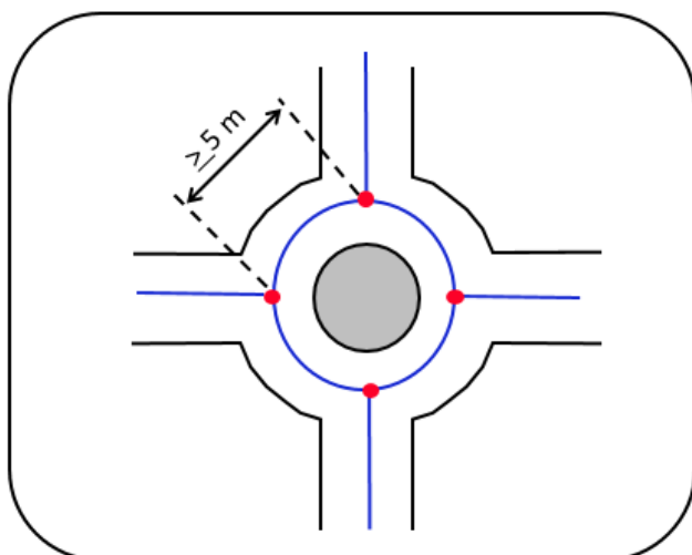
Figur 36 Cirkulationsplats (5 m gäller för avståndet mellan noder).
