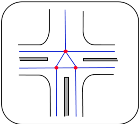
Figur 30 Två vägar med skilda körförhållanden och två utan. I dessa situationer kan det vara svårt att undvika snäva vinklar.
