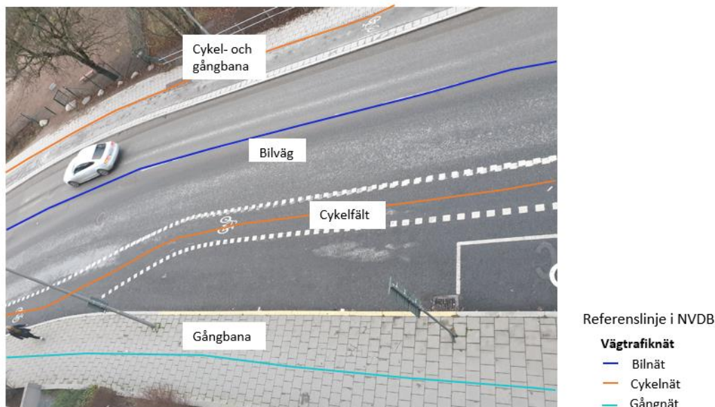
Figur 65 Exempel på när gång- och cykelbana ska delas upp i två separata referenslinjer på grund av fysisk avskiljare (typfall 6).
