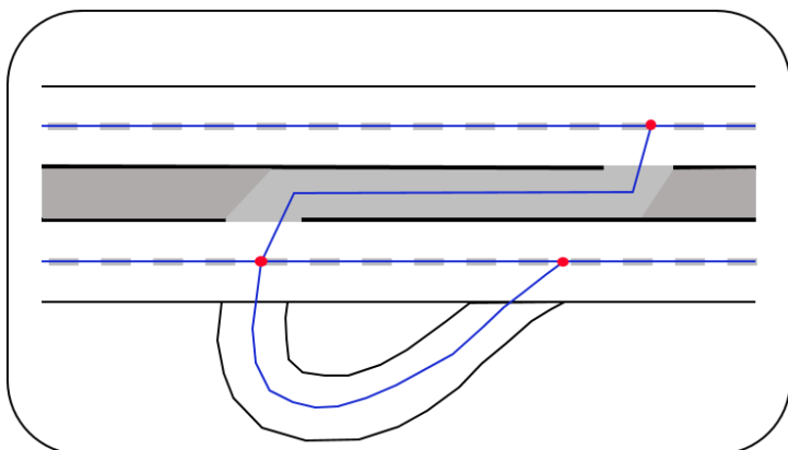
Figur 57 Exempel på driftvändplats där länken mellan vägbanorna måste anpassas efter fordonsrörelsen.
