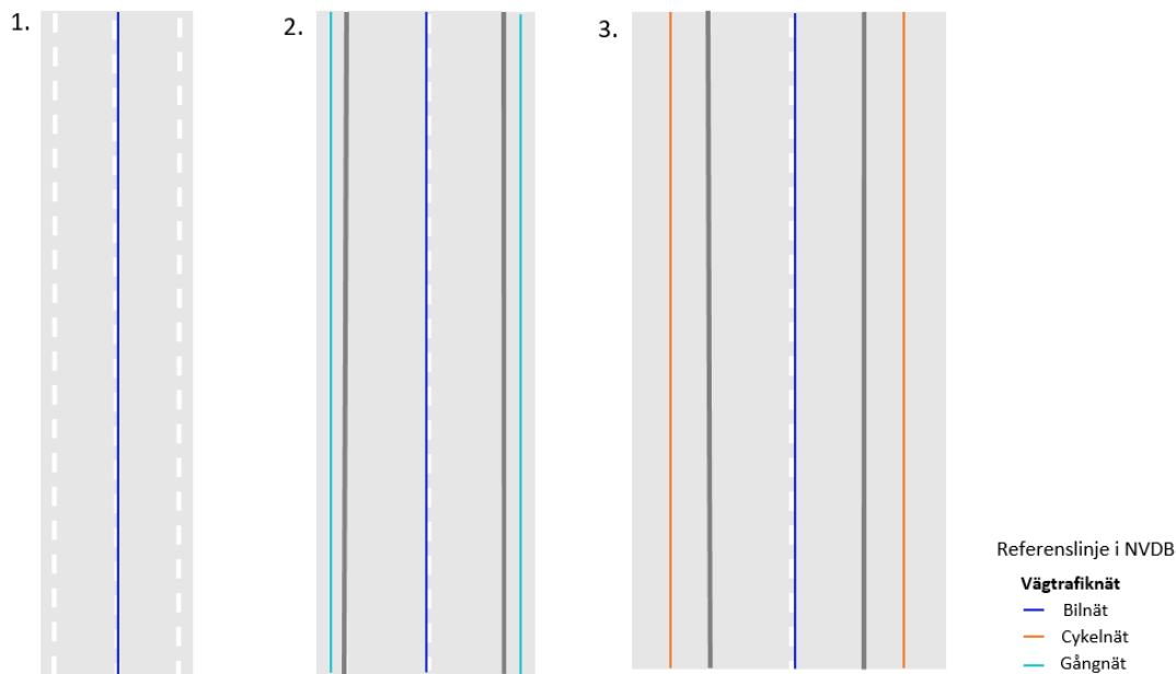
Figur 61 Illustration av typfall för avbildning av referenslinje för gång- och cykelnät.
