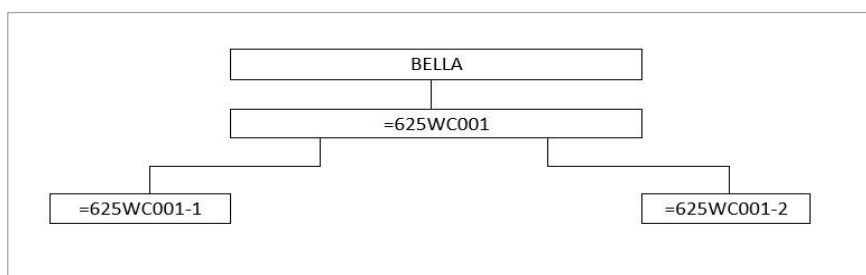
Figur 4.11.2-1 Kravprincip på elcentral med två anslutna grupper.
