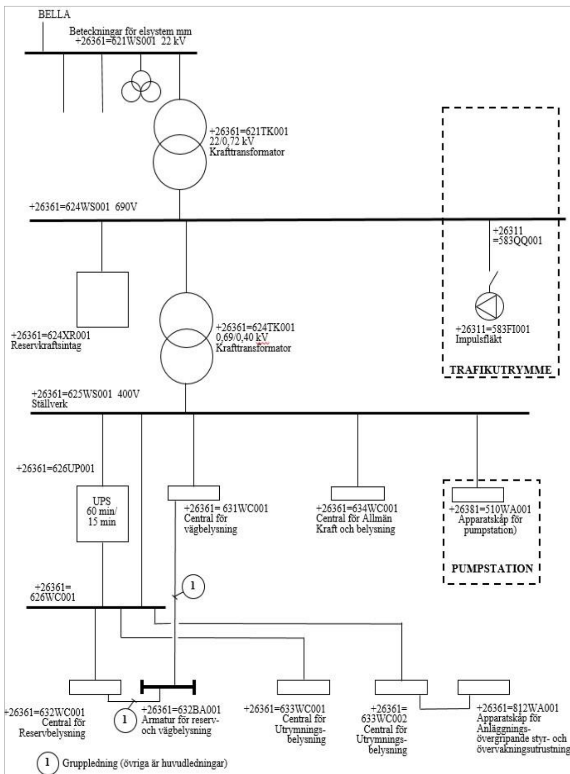
Figur 4.7.4-3 Kravprincip för systemhierarki för El i tunnel.
