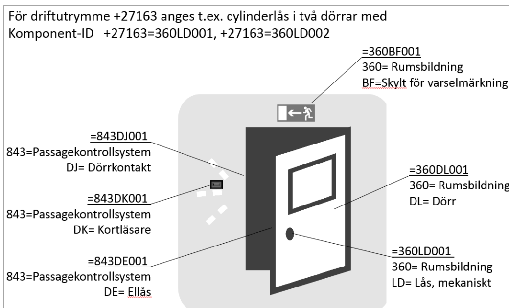
Figur 4.4.3 Kravprincip för dörrkomponenter.
