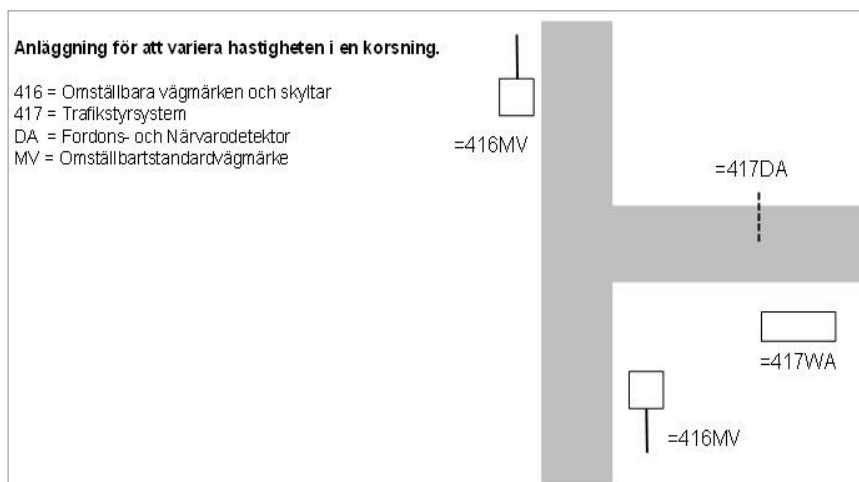
Figur 4.5.3.7. Kravprincip för korsning med varierande hastighet.
