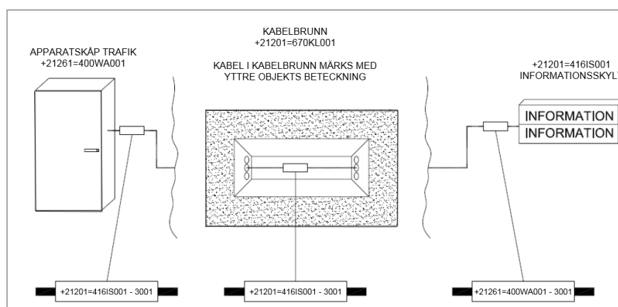
Figur 4.12.3 Kravprincip för kabelmärkning i kabelbrunn.
