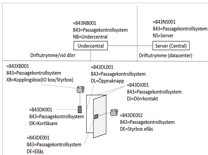
Figur 4.9.4.3 Kravprincip för Passersystem (843).
