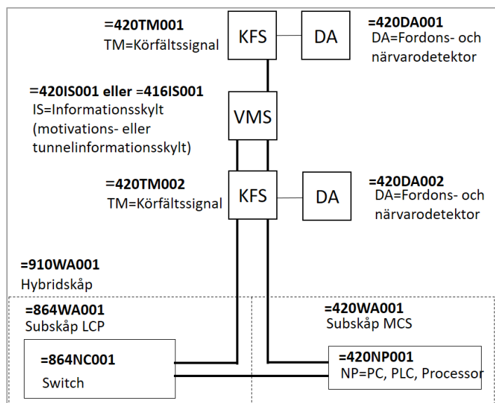
Figur 4.5.3.2-3. Kravprincip för MCS (ombyggd från MTM/2 till LASSY).
